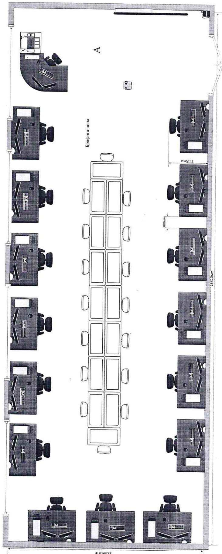
План застройки площадки ДЭ, проводимого в рамках ПУ с включением вариативной части Общая площадь площадки: 76,29 м2
